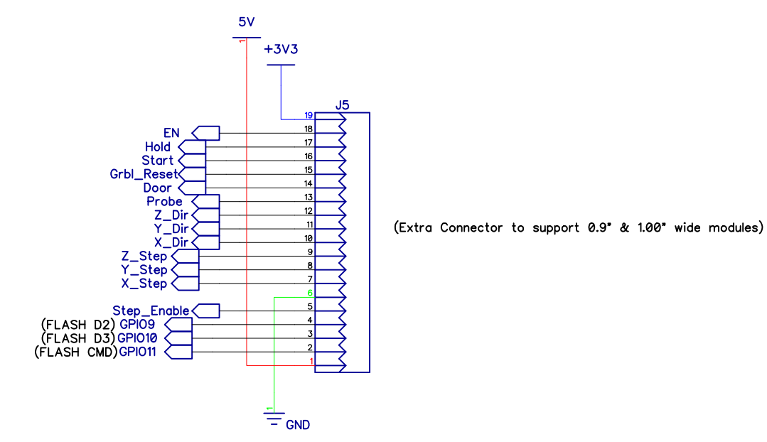
ESP32 Module
