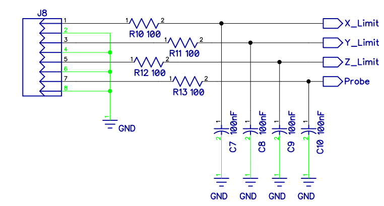
Inputs
